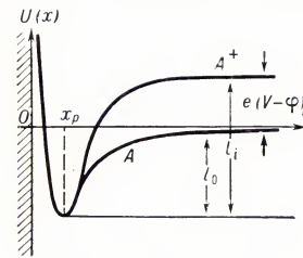
Рис. 1. Потенциальные кривые взаимодействия систем поверхность твердого тела — нейтральной частицы (A) и поверхность — положительный ион (A + ); x — удаление от поверхности; U(x) — энергия связи частицы с поверхностью. Расстояние x_p соответствует равносному состоянию частицы у поверхности, а глубины «потенциальных ям» l_i и l_0 равны теплотам десорбции иона и нейтральной частицы соответственно. Разность l_i - l_0 в данном случае равна разности энергии ионизации eV нейтральной частицы ( V — её ионизационный потенциал, e — заряд электрона) и работы выхода поверхности e\phi .
